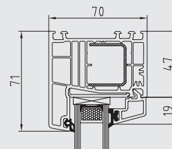
Oberlicht Fest
