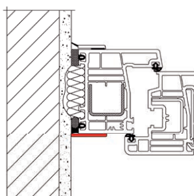
Flachleiste selbstklebend
