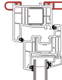
Rollladenablaufprofil R1 und Rollladendeckelaufnahmeprofil R2
