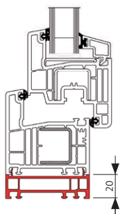
Verbreiterungsprofil
