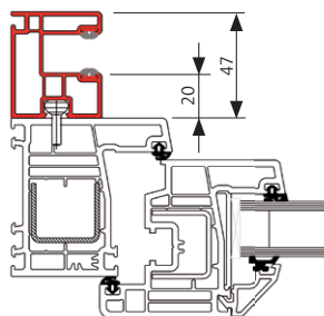
Rollladenführungsschiene R 110 K
