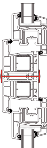
Kopplungsprofil
