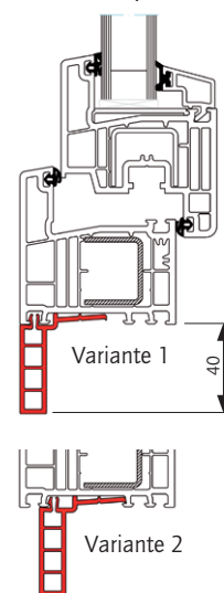
Fensterbank- anschlussprofil V7
