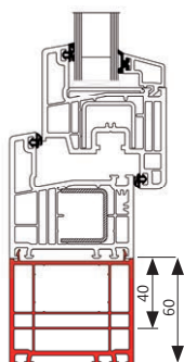
Verbreiterungsprofil
