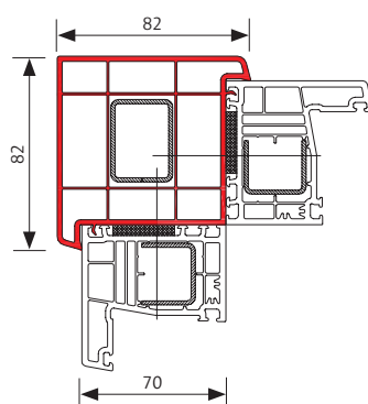
Eckverbinder 90° K 238
