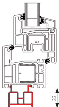
Fensterbank- anschlussprofil V13
