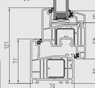
Fenster 1-flügelig, Dreh-Kipp
