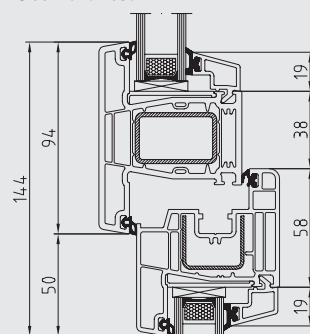
Fenster 1-flügelig, Dreh-Kipp
