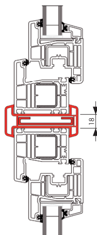
Kopplungsprofil
