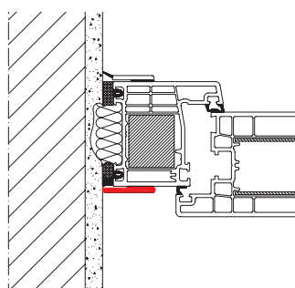
Flachleiste selbstklebend
