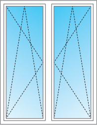
Balkontüren 2-flg., symmetrisch, Dreh-Kipp/Dreh-Kipp, fester Pfosten
