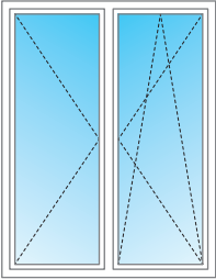
Balkontüren 2-flg., symmetrisch, Dreh/Dreh-Kipp, Stulp
