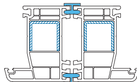
Kopplungsprofil G 3284
