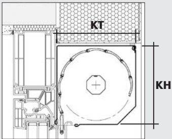
Vorbau-Rollladen eckiger Kasten mit 45°-Schräge in Laibung eingebaut
