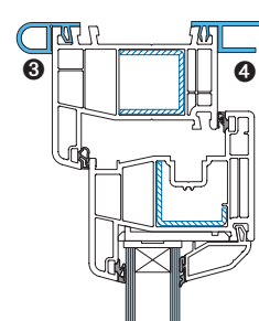
Rollladenabrollprofil G 3342 ③ und Rollladendeckel- aufnahmeprofil G 3345 ④
