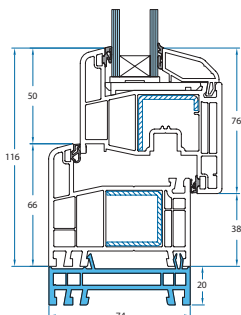
Verbreiterungsprofil G 2315
