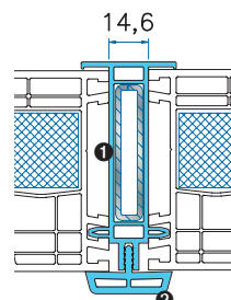
Kopplungs-Statikprofil ① = G 7281/7791 Abdeckung ② = G 3292
