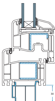
Fensterbankanschluss- profil G 7202
