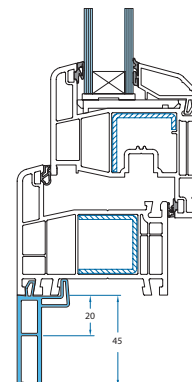
Fensterbankanschluss- profil, Altbau, G 3216
