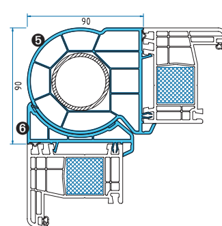
Eckverbinder variabel Rundprofil 2233 ⑤ / Adapter 2233 ⑥
