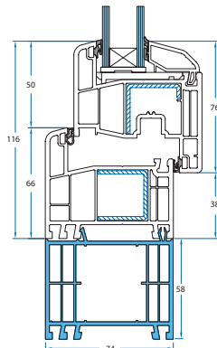
Verbreiterungsprofil G 7292
