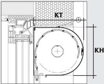
Vorbau-Rollladen runder Kasten in Laibung eingebaut
