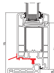
Wetterschenkel (ALU) mit Bürstendichtung und Befestigungsschrauben
