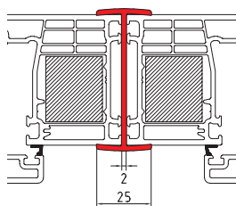
Kopplungsprofil PAD 60 / K3
