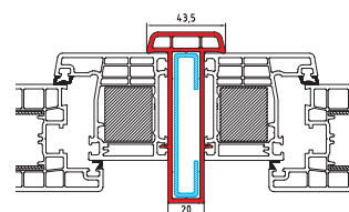
Kopplungs-Statikprofil A-K6070 / K223
