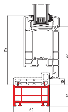
Blendrahmenverbreiterung PAD 60 / V3 auch verwendbar als Bodeneinstandsprofil 35 mm (V3)
