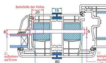
Kopplungsprofil G 3284
