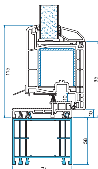
Verbreiterungsprofil G 7292 58 mm ( unter Bodenschwelle )
