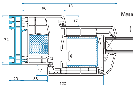
Fensterbankanschlussprofil G 3216
