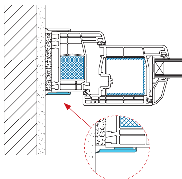
Flachleiste selbstklebend
