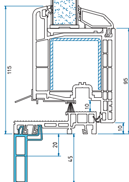
Flachleiste selbstklebend
