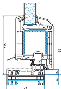
Verbreiterungsprofil G 2315 20 mm ( unter Bodenschwelle )
