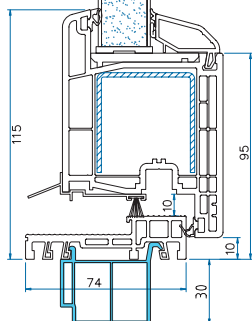
Fensterbankanschlussprofil G 7202
