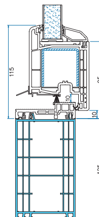
Bodeneinstandsprofil G 2311 125 mm
