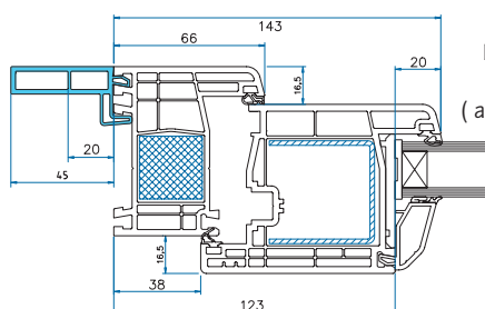
Maueranschlussprofil G 2315 20 mm ( am Rahmen seitlich )
