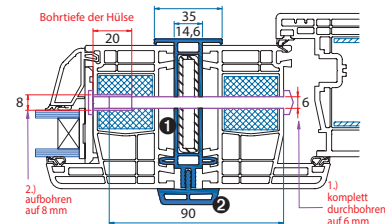
Kopplungs-Statikprofil G 7281/7791 1 Abdeckung 2 = G 3292
