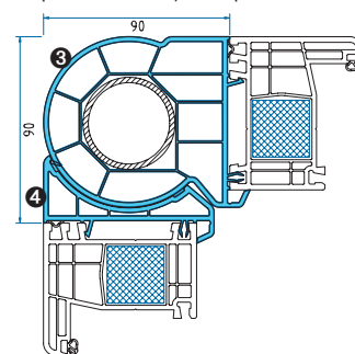
Eckverbinder variabel Rundprofil 2233 3 / Adapter 2233 4
