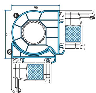
Eckverbinder variabel Rundprofil 2233 ⑤ / Adapter 2233 ⑥
