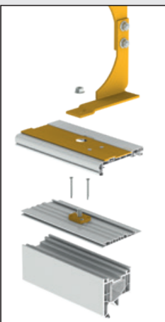
Blendrahmenstabilisierung TOP MINI plus RvU
